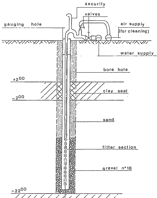
Fig. 3 : Berendrecht : Recharge well
