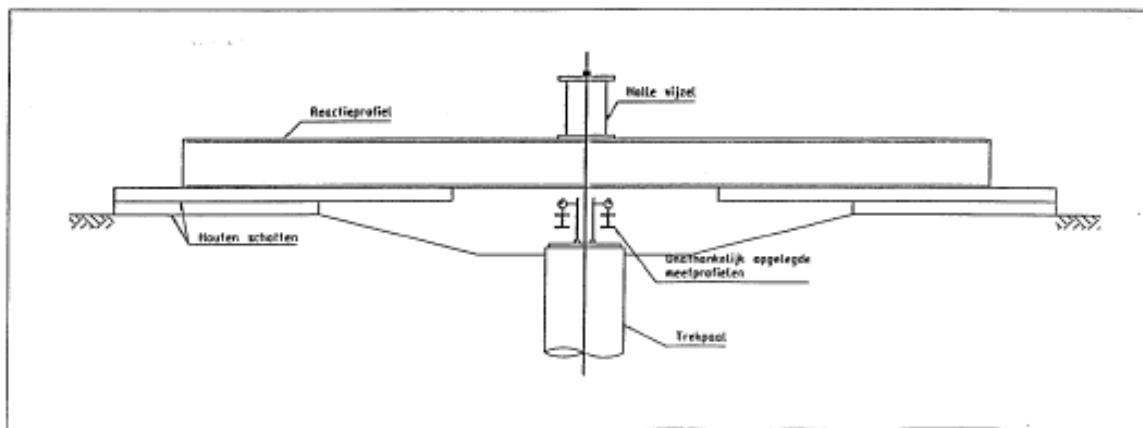
Fig 3b : Principeschets trekproef
