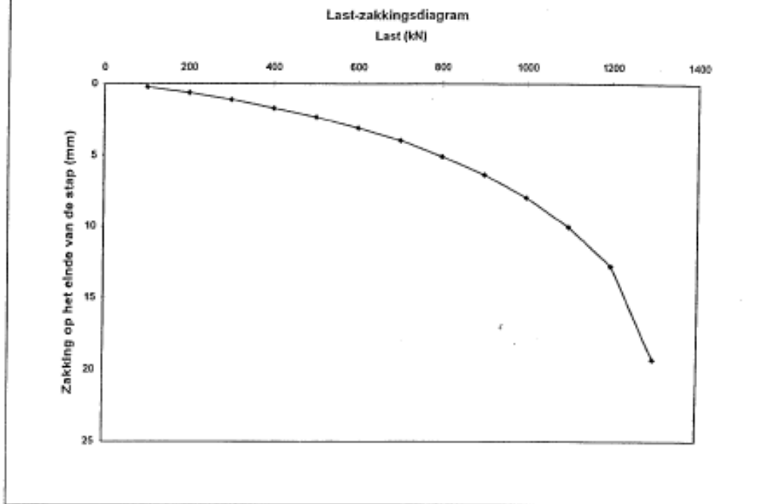
Fig. 4c : Interpretatie van de belastingsproef - Trekproef - Paal 1
