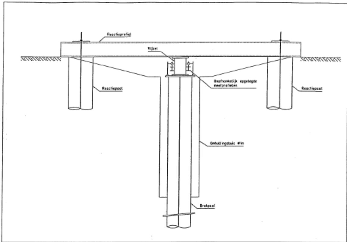
Fig 3a : Principeschets drukproef
