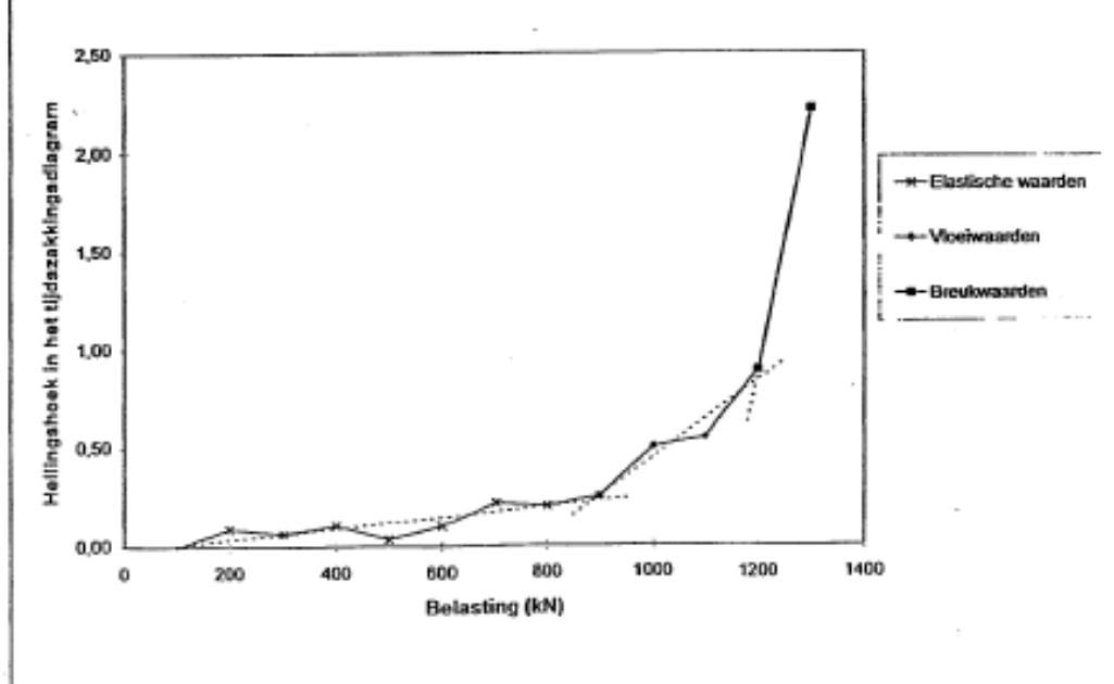
Fig. 4b : Interpretatie van de belastingsproef - Trekproef - Paal 1 Last-hellingsdiagram
